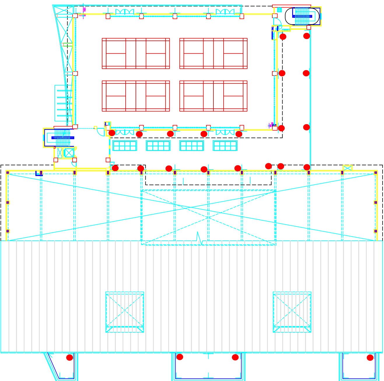
參層，參層夾層及屋突壹層平面圖
